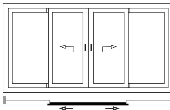
Čtyřdílné, schéma C
